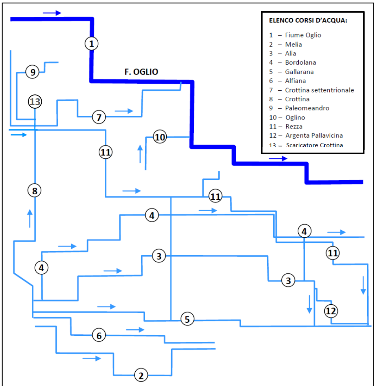
Schema Idrografico – Comune di Bordolano
